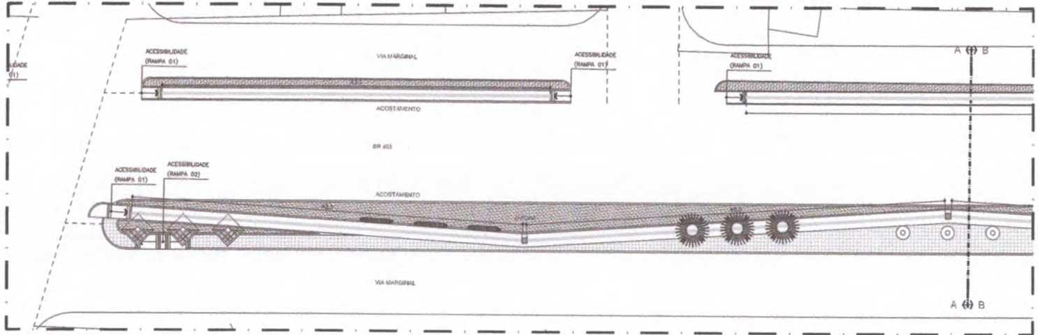
30.01 PLANTA BAIXA - ACESSIBILIDADE TRECHO 02/A ESCALA 1:250
