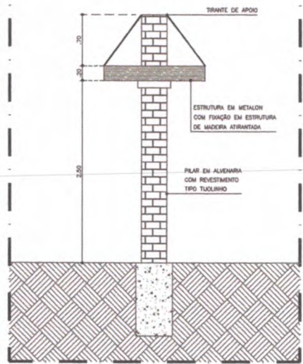
17.05 VISTA - CARAMANCHÃO 02 ESCALA 1:20
