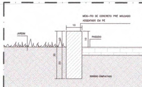
16.05 | DETALHE - MEIO FIO 02 ESCALA 1:50
