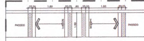
29.04 RAMPA 02 - PLANTA BAIXA ESCALA 1:50
