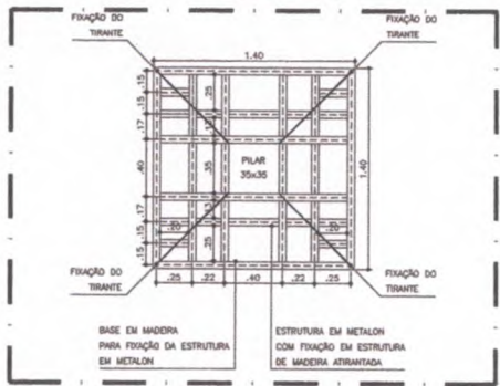
17.03 PLANTA BAIXA - CARAMANCHÃO 02 ESCALA 1:20
