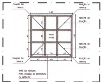
17.04 DETALHE - SUPORTE CARAMANCHÃO 02 ESCALA 1:20
