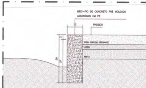
16.04 | DETALHE - MEIO FIO 01 ESCALA 1:50
