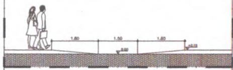
35.05 | RAMPA 02 - VISTA ESCALA: 1/50
