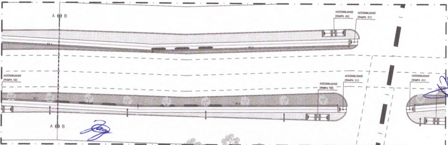
33.02 PLANTA BAIXA - ACESSIBILIDADE TRECHO 05/B ESCALA 1/200
