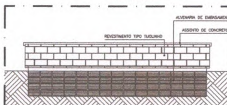
16.11 | CORTE - BANCO RETO ESCALA 1:25
