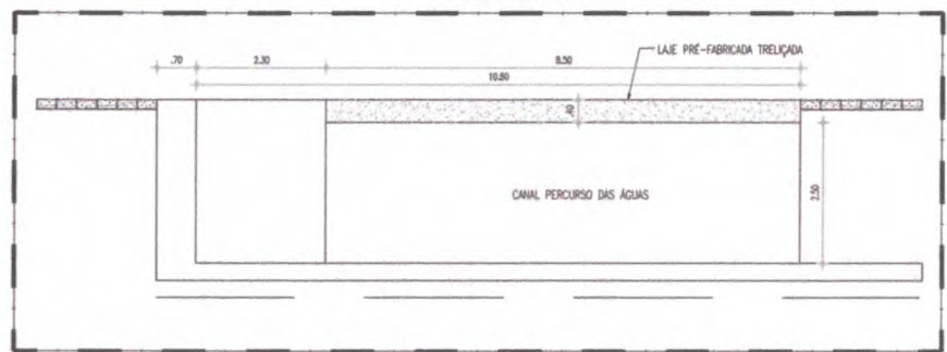
39.02 | CORTE LONGITUDINAL AA ESCALA 1:50
