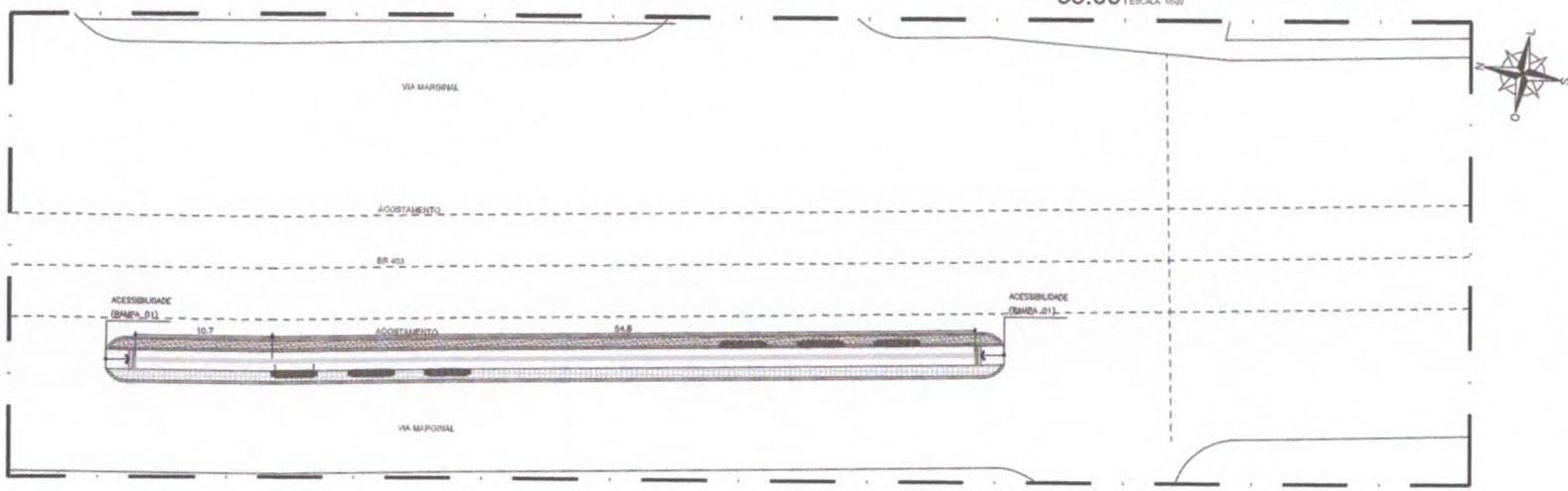
35.01 | PLANTA BAIXA - ACESSIBILIDADE TRECHO 07A ESCALA: 1/200
