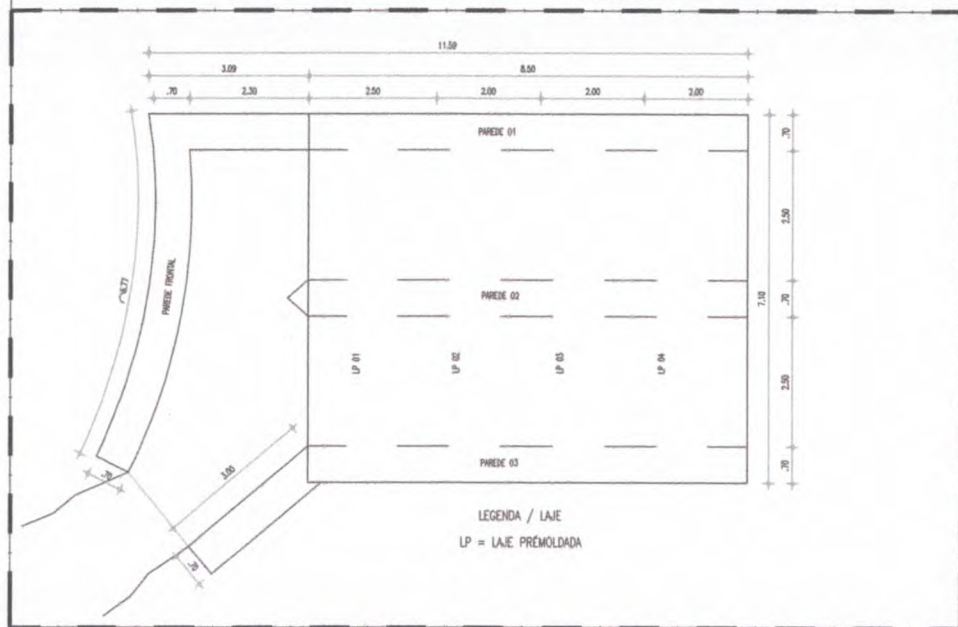
38.01 | LEGENDA LAJE ESCALA 1:50
