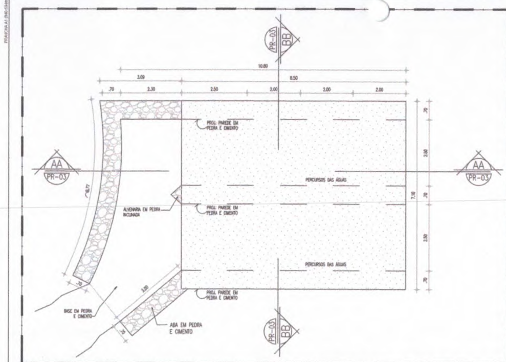
38.00 | PLANTA BAIXA - AMPLIAÇÃO DO SANGRADOURO ESCALA 1:50
