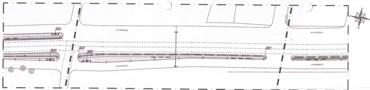
34.00 | PLANTA BAIXA - ACESSIBILIDADE TRECHO 06 ESCALA 1/250
