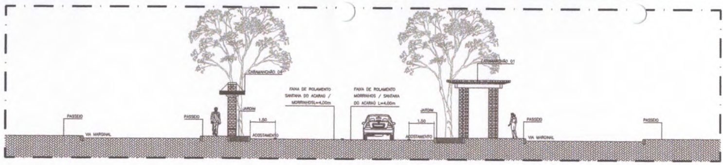
18.00 | CORTE TRECHO 01 ESCALA 1/15
