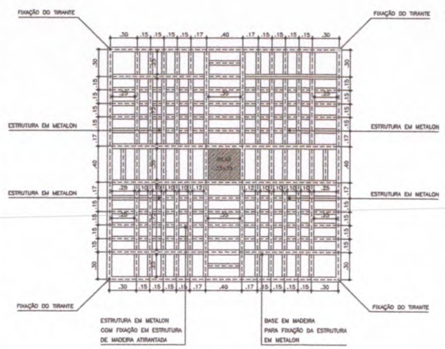
17.00 PLANTA BAIXA - CARAMANCHÃO 03 ESCALA 1:20
