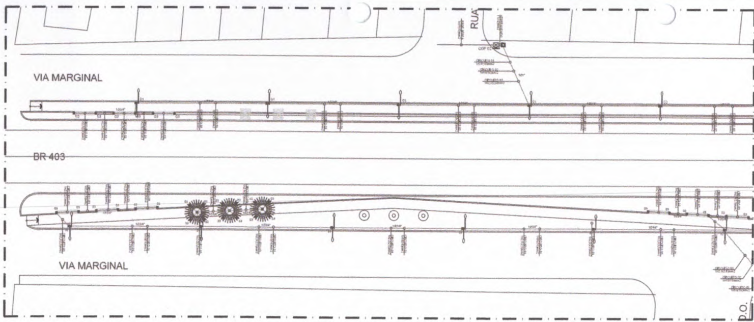
20.00 | PLANTA BAIXA - ELÉTRICA TRECHO 01.01 ESCALA 1/300
