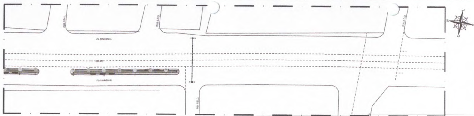
35.00 | PLANTA BAIXA - ACESSIBILIDADE TRECHO 07 ESCALA: 1/500
