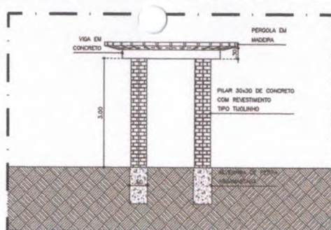
16.01 | VISTA 01 - CARAMANCHÃO 01 ESCALA 1:50
