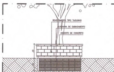
16.08 | JARDINEIRA - DETALHE 02 ESCALA 1:25
