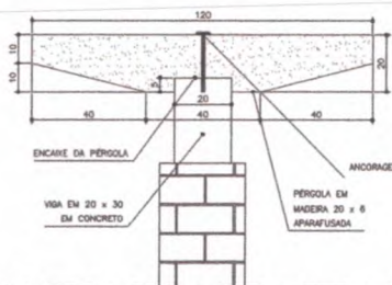
16.03 | DETALHE - PÉRGOLA ESCALA 1:50
