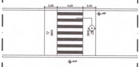
17.07 DETALHE - TRAFIC CALMING ESCALA 1:12.5
