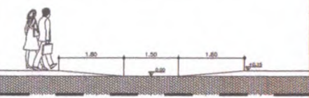
34.05 | RAMPAS 02 - VISTA ESCALA 1/50
