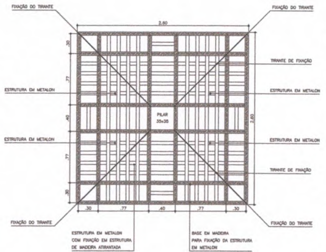
17.01 DETALHE - SUPORTE CARAMANCHÃO 03 ESCALA 1:20
