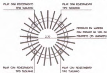
16.00 | PLANTA BAIXA - CARAMANCHÃO 01 ESCALA 1:50
