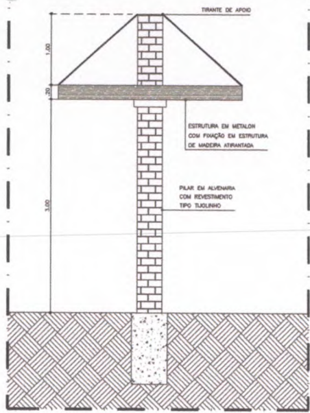
17.02 VISTA - CARAMANCHÃO 03 ESCALA 1:20
