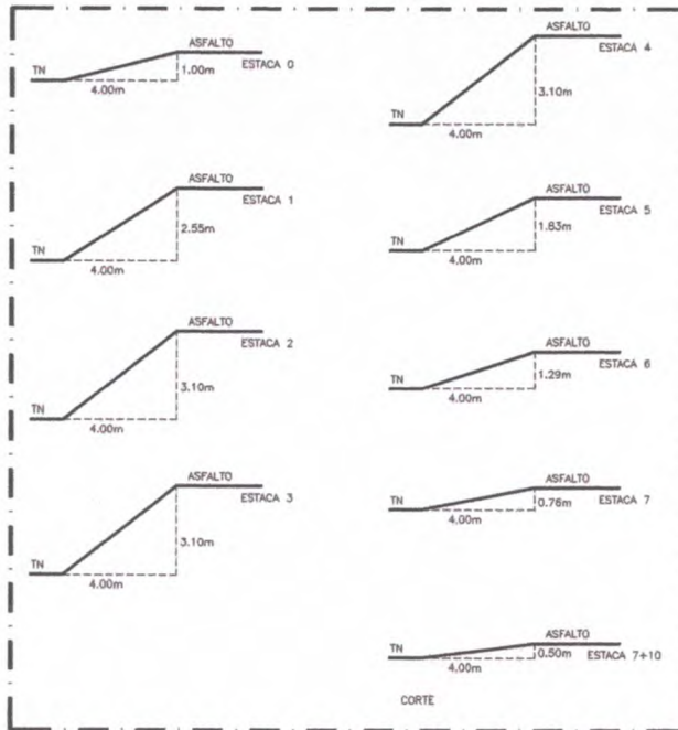
37.02 | CORTE TRECHO 04 ESCALA 1/10
