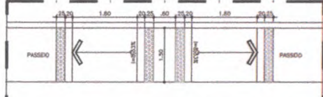
35.04 | RAMPA 02 - PLANTA BAIXA ESCALA: 1/50
