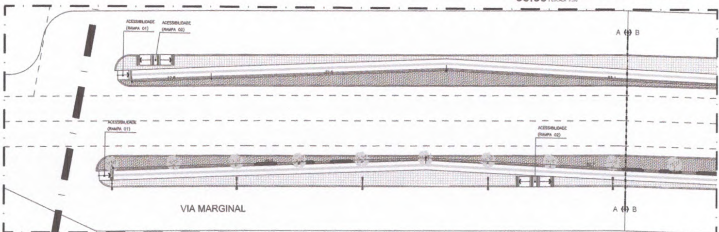
33.01 PLANTA BAIXA - ACESSIBILIDADE TRECHO 05/A ESCALA 1/200
