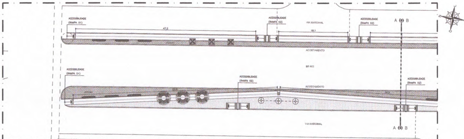
29.01 PLANTA BAIXA - ACESSIBILIDADE TRECHO 01/A ESCALA 1:200
