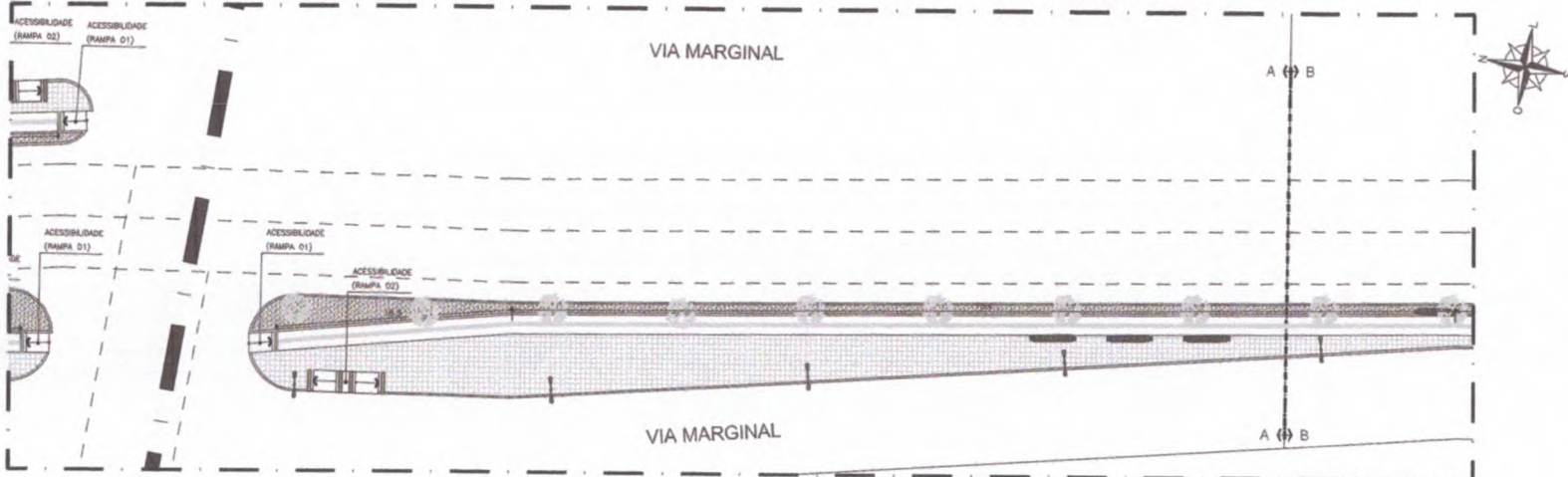
34.01 | PLANTA BAIXA - ACESSIBILIDADE TRECHO 06/A ESCALA 1/250
