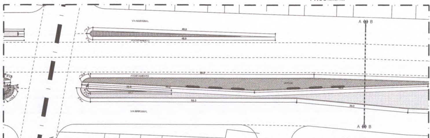
11.01 PLANTA BAIXA - IMPLANTAÇÃO TRECHO 03/A ESCALA 1/250
