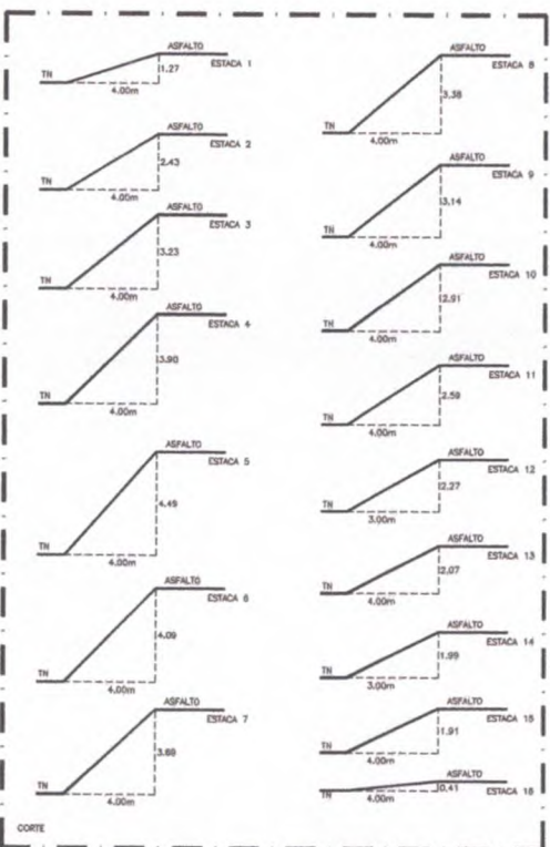
36.02 | CORTE TRECHO 04 ESCALA: 1/50
