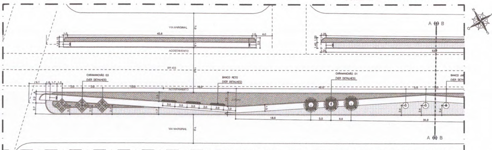
03.01 | PLANTA BAIXA - IMPLANTAÇÃO TRECHO 02/A ESCALA 1:250
