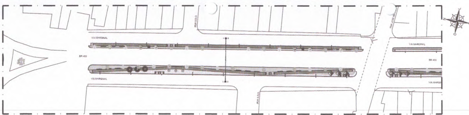
29.00 PLANTA BAIXA - ACESSIBILIDADE TRECHO 01 ESCALA 1:500
