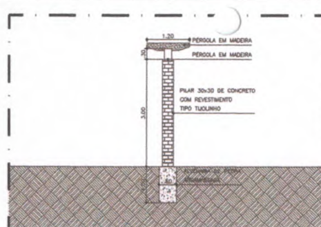
16.02 | VISTA 02 - CARAMANCHÃO 01 ESCALA 1:50
