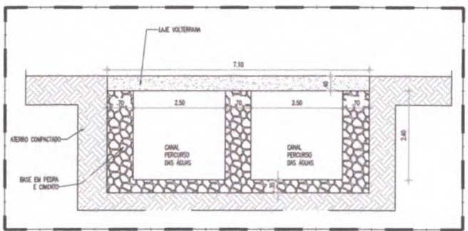
39.01 | CORTE TRANSVERSAL BB ESCALA 1:50
