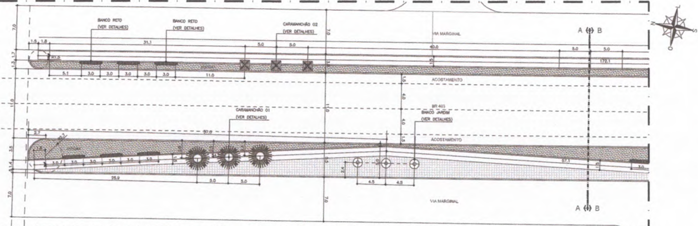
02.01 PLANTA BAIXA - IMPLANTAÇÃO TRECHO 01A ESCALA 1:200
