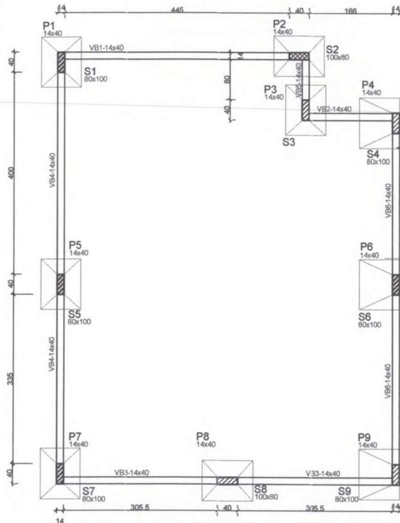
Forma Fundações escala 1:50
